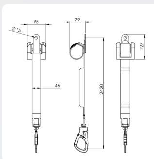
ENCOMBREMENT
